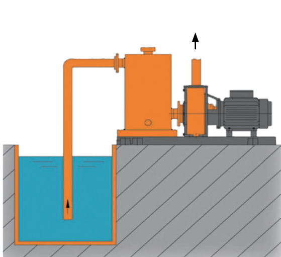
Operazione di aspirazione Svuotamento fossa
