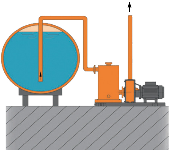
Funzionamento ad aspirazione Svuotamento caldaia
